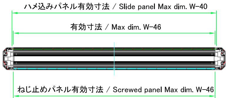
A-A ( 1 : 5 )
