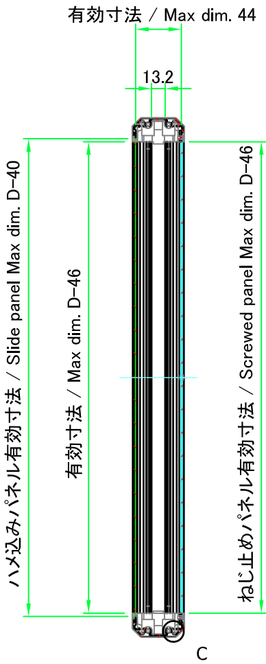
B-B ( 1 : 5 )
